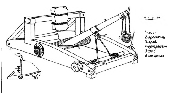
Сл. 3. ПРЕТПОСТАВЕН ИЗГЛЕД НА ФРЛАЧКАТА ПОСТРОЈКА - СКОРПИОН
